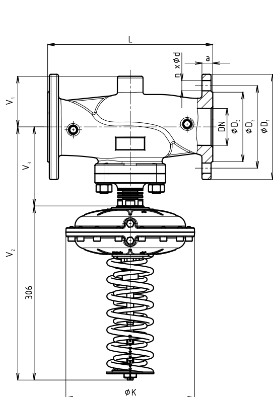
Исполнение RD 212 D (камера 240 см 3 )
