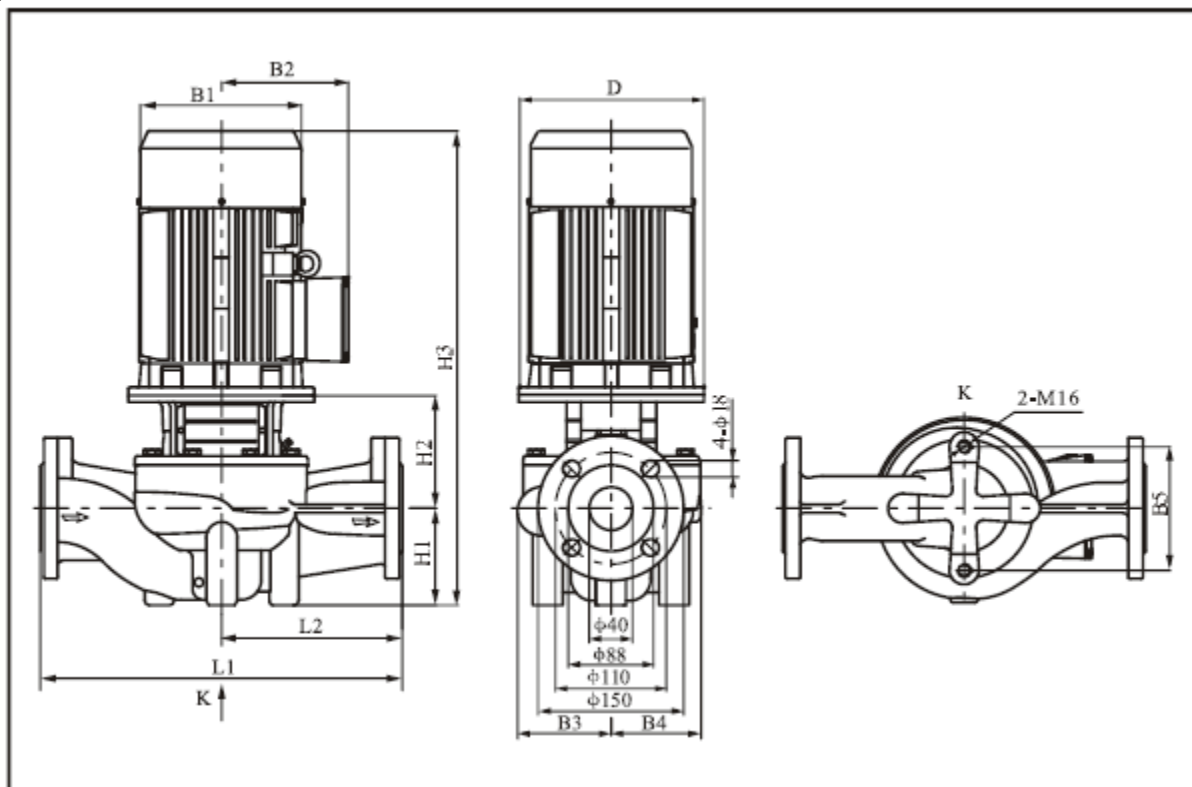
Схема установки
