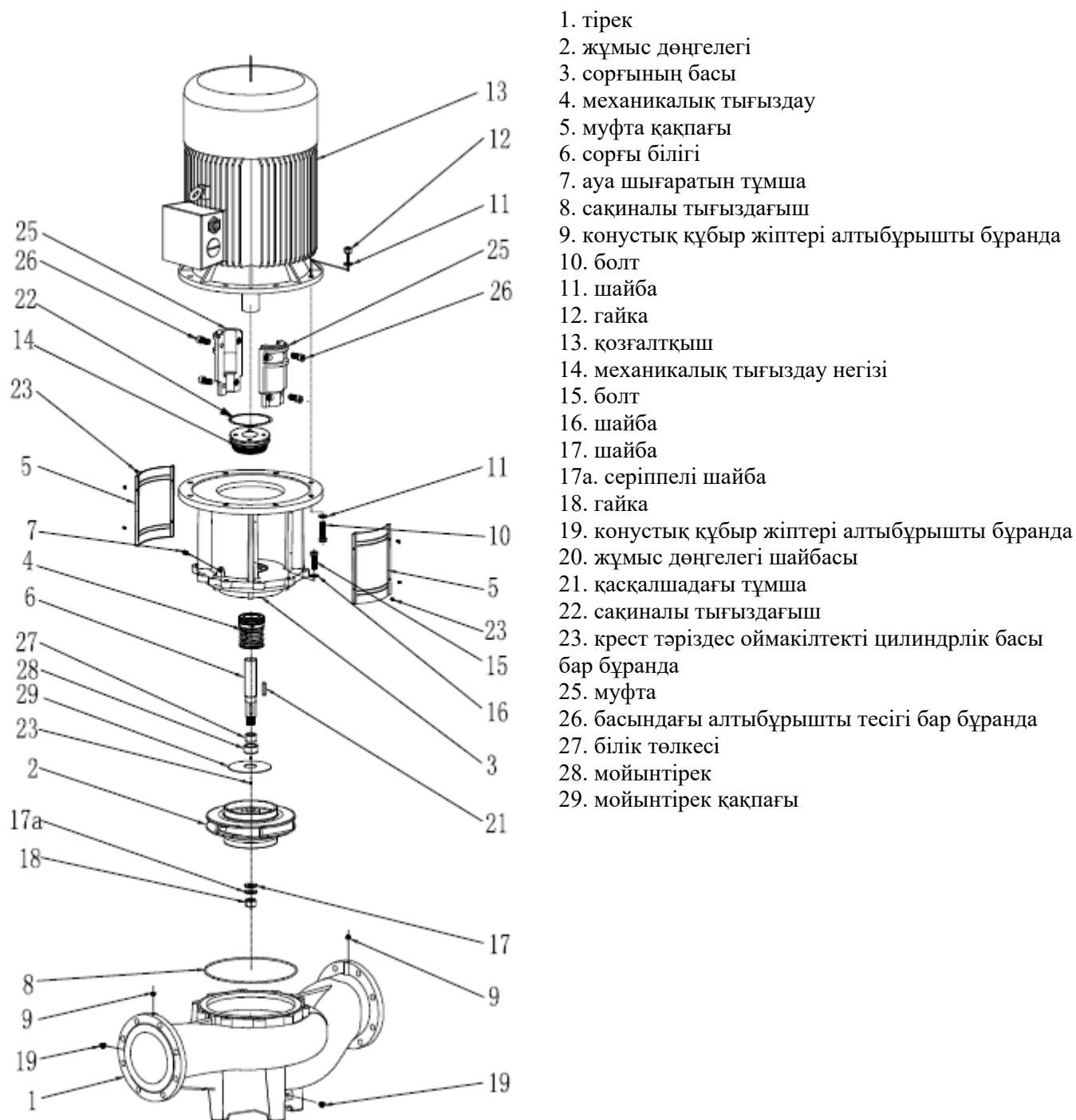
TK125-18/4-TK150-50/4-160301 Оңай жиналатын құралым
