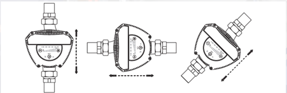
Сорғы білігінің рұқсат етілген қалпы
