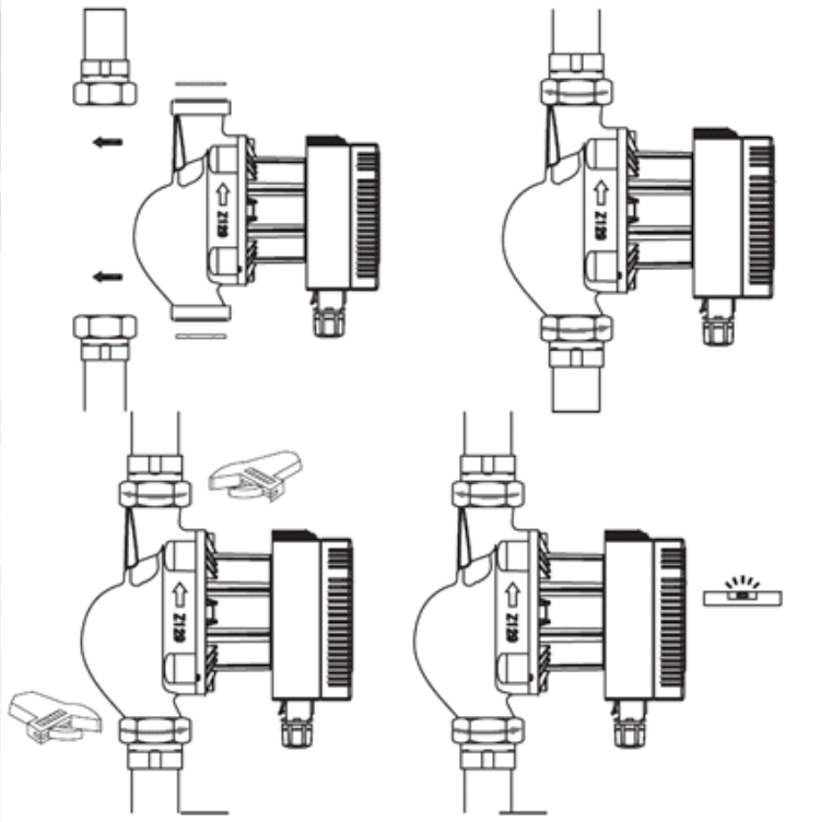
Сорғыны орнату
