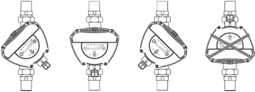
MEGA сорғысының электрондық блогының орналасу схемасы
