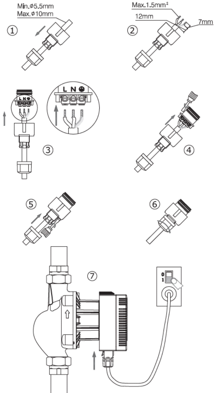
MEGA сорғысының электр қосылымы
